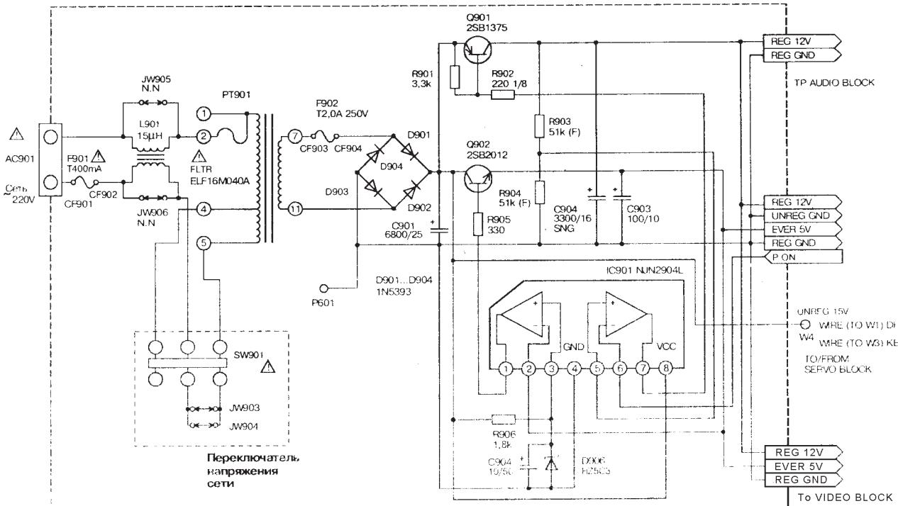
Принципиальная схема источника питания видеоплеера HV-E295DK.
